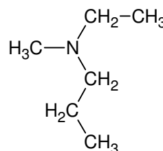
N -éthyl, N -méthylpropanamine
